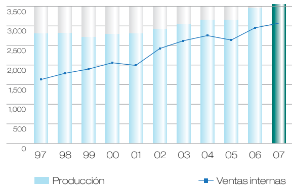
Producción y ventas internas de gas seco millones de pies cúbicos diarios
